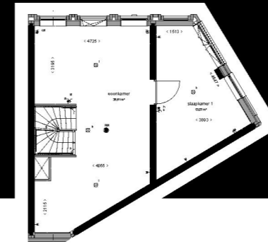
EERSTE VERDIEPING
