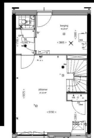
BEGANE GROND
