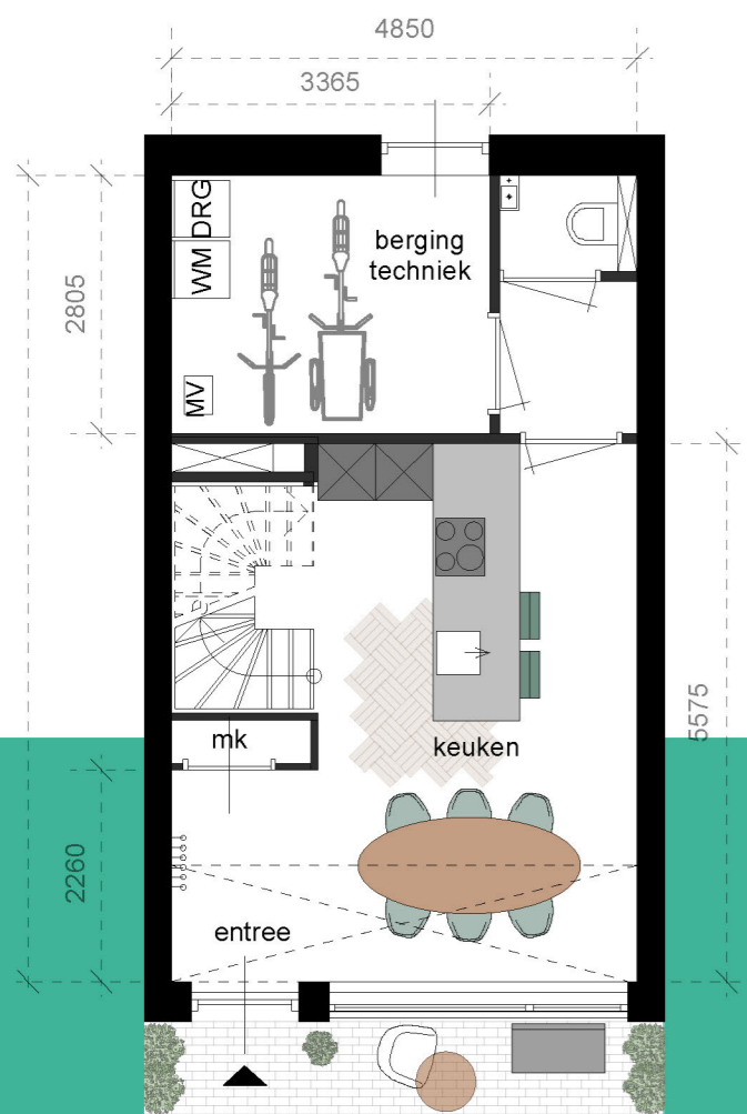
BEGANE GROND
