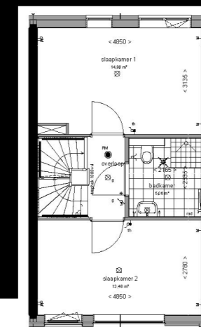
TWEDE VERDIEPING
